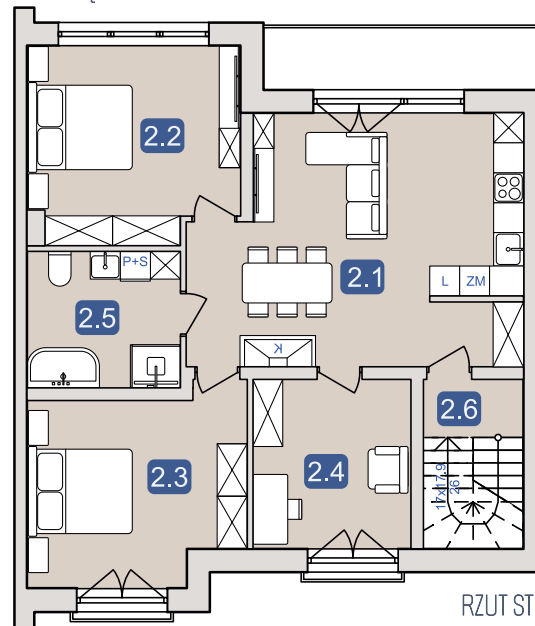
RZUT PIĘTRA
